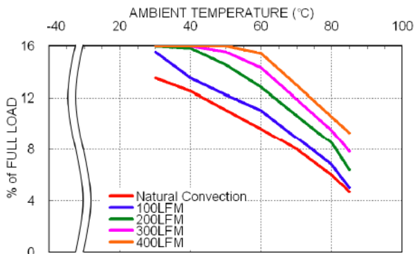
POLS16-05T, Vout=3.3V Derating Curve
